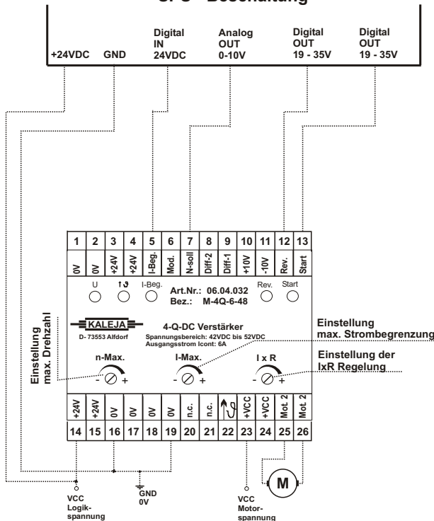
SPS - Beschaltung
