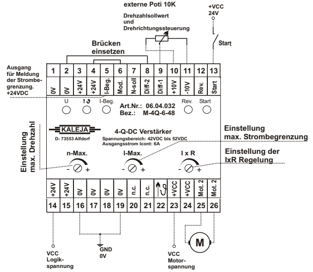
Differenzeingang-Beschaltung
