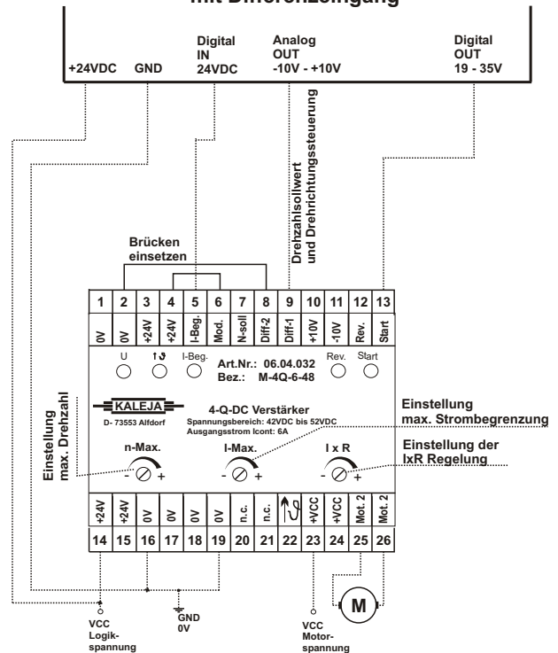
SPS - Beschaltung mit Differenzeingang
