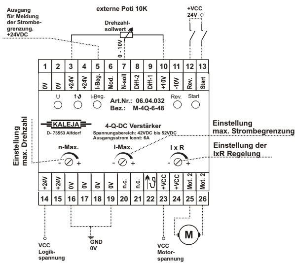
Standard - Beschaltung
